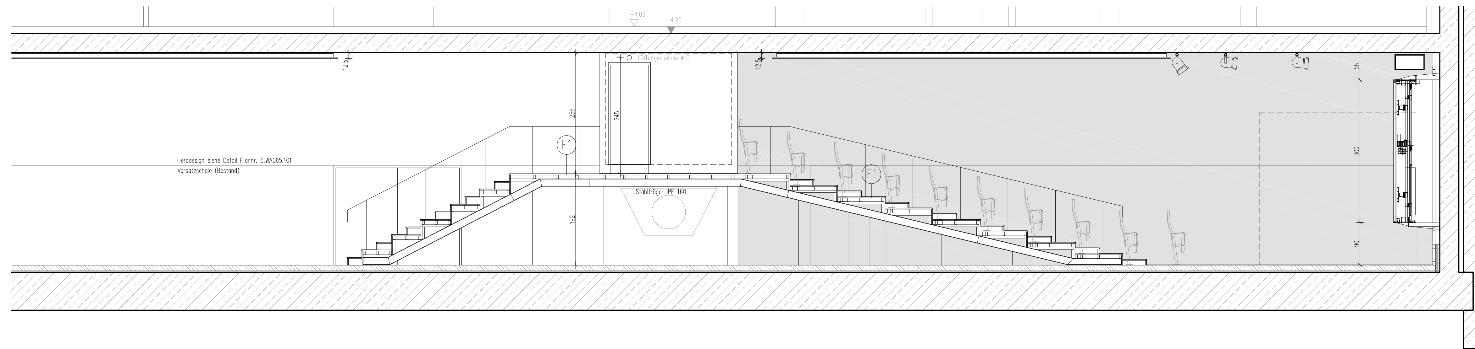
Schnitt B-B 1:50
