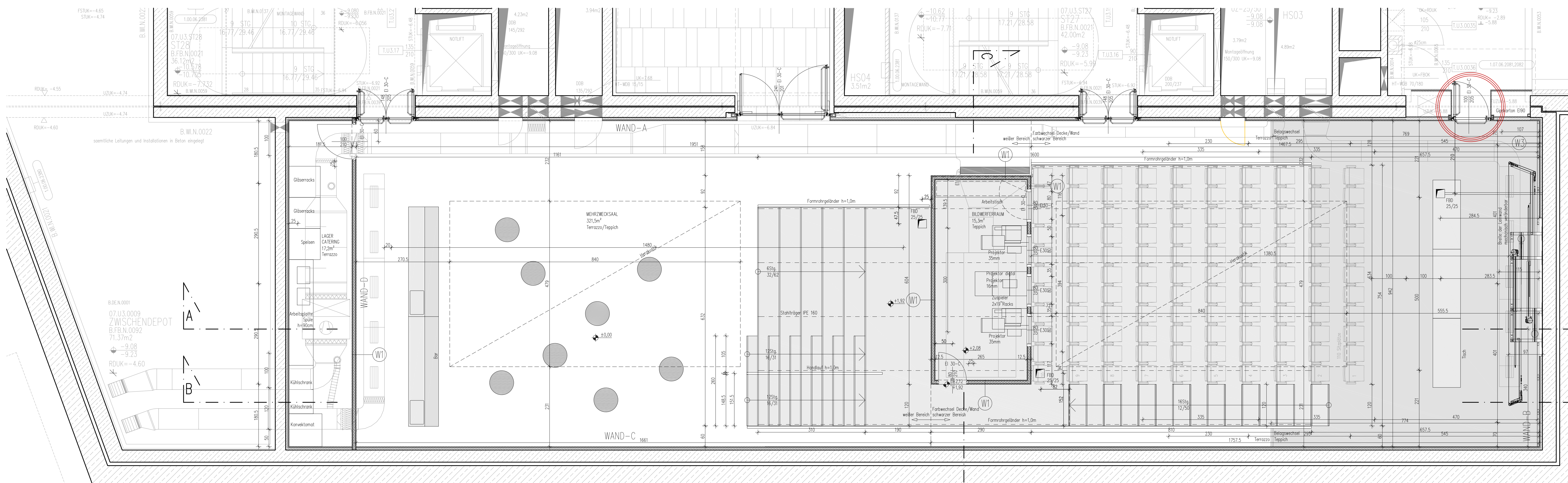
GRUNDRISS 1:50
