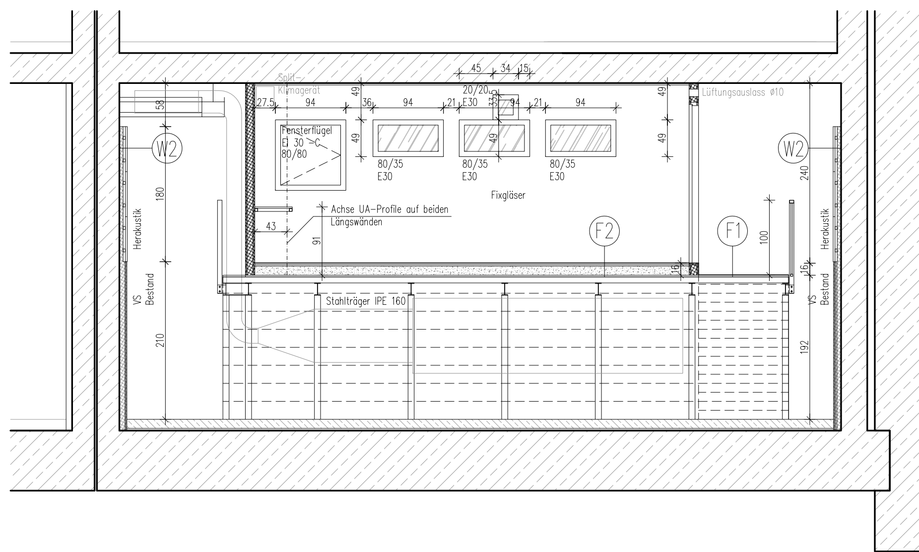
Schnitt C-C 1:50
